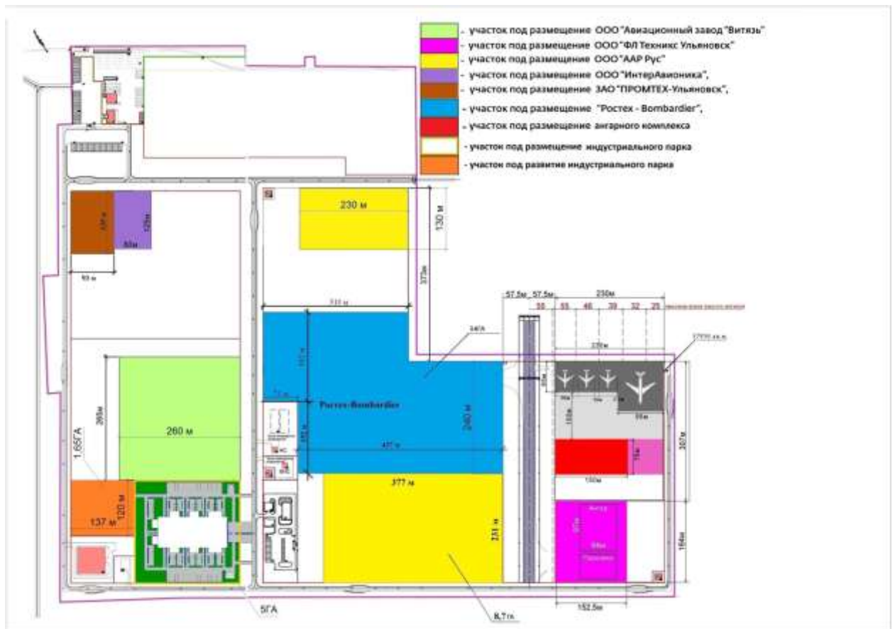
Рис. 1.2. Схема размещения объектов на территории ПОЭЗ (1-й пусковой комплекс)
